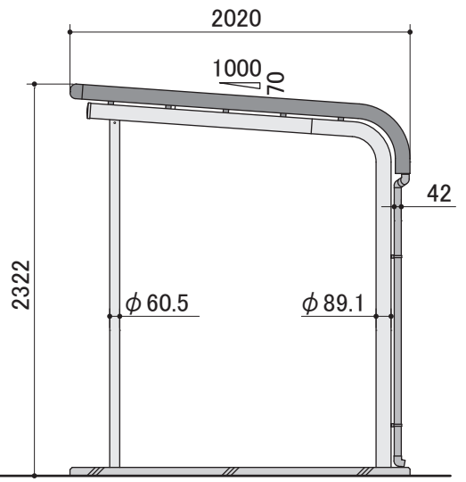
側面図
